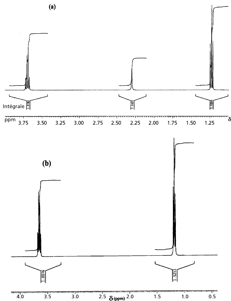
Figure 4.14 Spectre de l'éthanol (a) dans CDCl 3 et (b) dans D 2 O.
