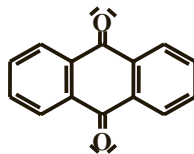
antraquinone
