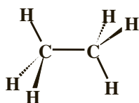
Conformation décalée
