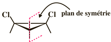
cis
