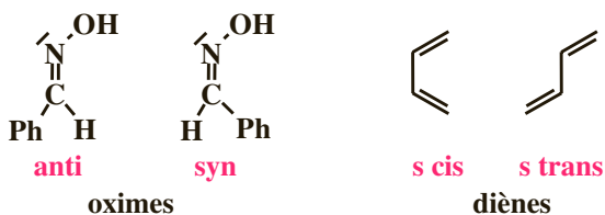
Figure 2.24 Exemples d'isométrie géométrique dans les oximes et dans les diènes.
