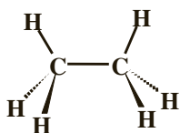
Conformation éclipsée
