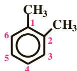
orthoxylyène (1,2-diméthylbenzène)
