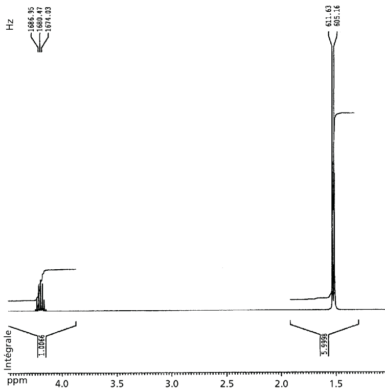
Figure 4.13 Spectre de RMN du 2-chloropropane ( \text{CH}_3\text{-CHCl-CH}_3 ).
