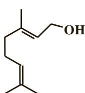
géraniol
