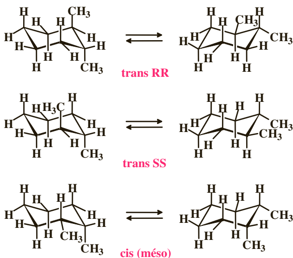
Figure 2.28 Cyclohexanes disubstitués-1,2.
