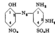
Chrome brown R (Kalle)
